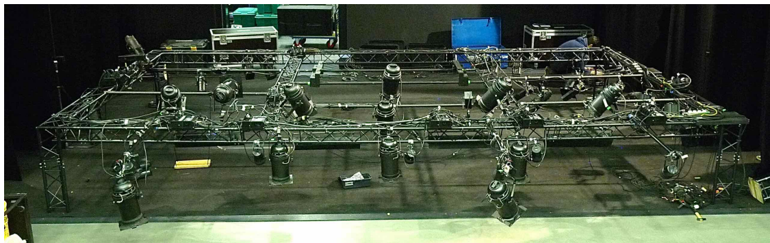
(Structure équipée avant levage)
